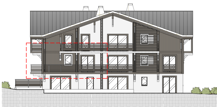
Façade Est
